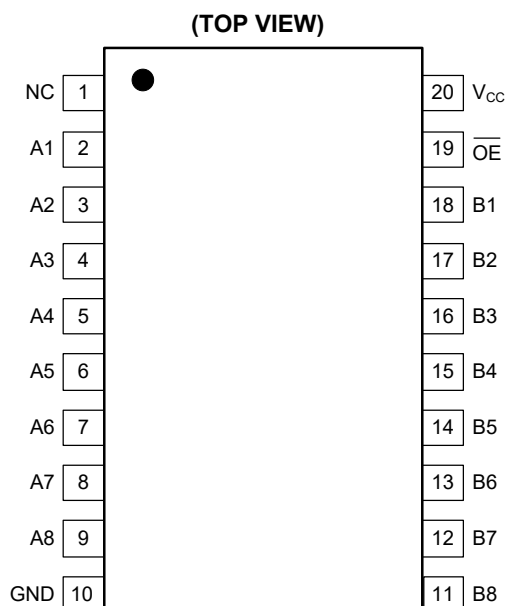
TSSOP-20
