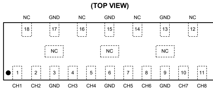
UTDFN-5.5 \times 1.5-18L
