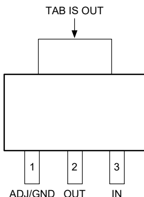
SOT-223-3
