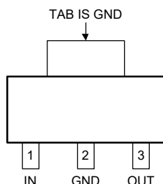
SOT-223-3
