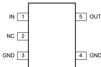
SOT-23-5
